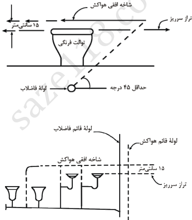
شکل شماره (۱۶-۶-۲-۵) "پ" (۲): اتصال هواکش به شاخه افقی لوله فاضلاب
