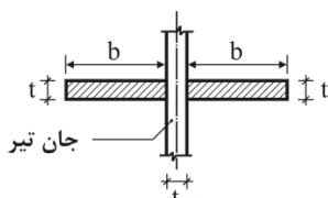
شکل ۱۰-۲-۶-۱ مقطع سخت‌کننده‌های عرضی
