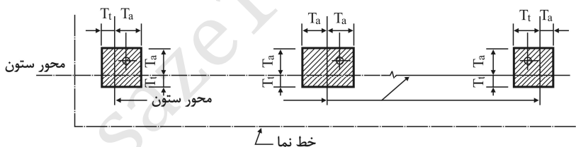
شکل ۱۱-۴-۱۰ ناريسماني ستون‌های داخلی
