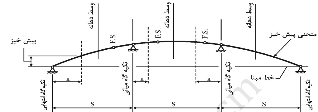
وصله کارگاهی F.S.
