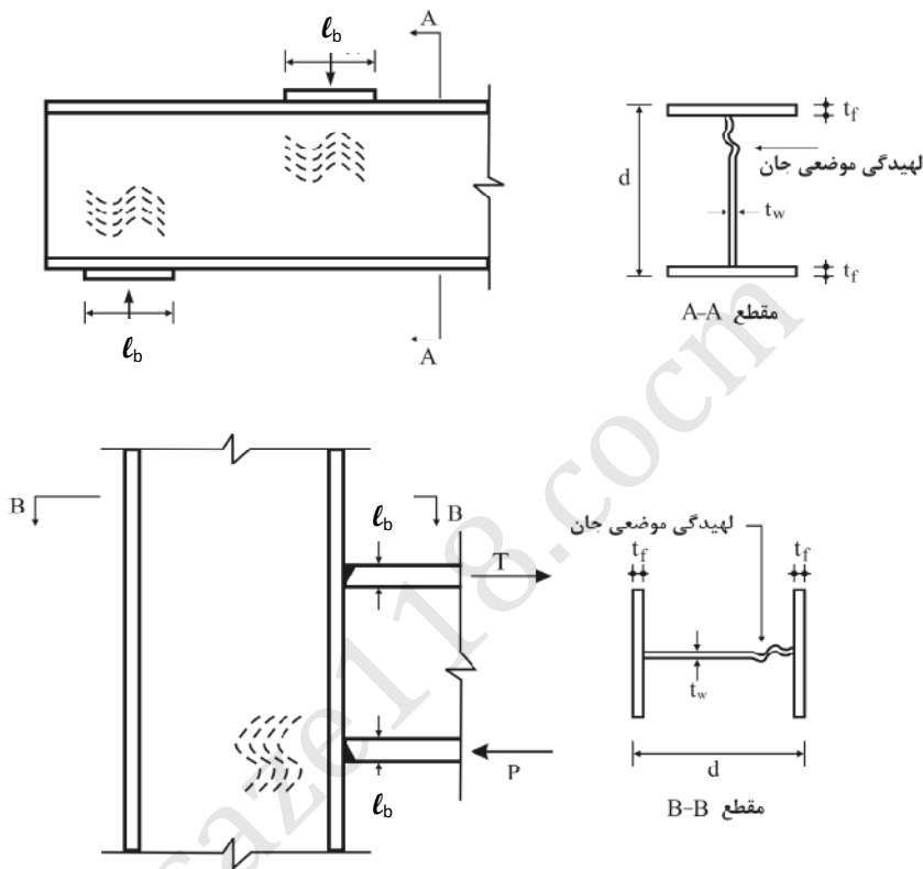
شکل ۲-۱۰-۹-۱۸ لپیدگی جان در مقابل نیروی متمرکز فشاری
