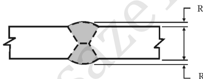
ورق ها با ضخامت مساوی
