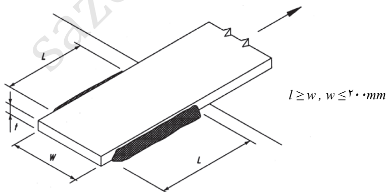
شکل ۱۰-۲-۹-۴ جوش گوشه در انتهای تسمه‌های کششی
