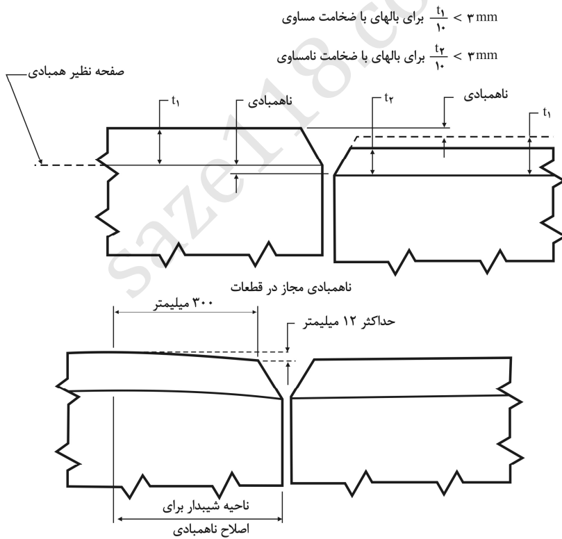
شکل ۴-۱۰-۲ اصلاح ناهمبادی و ناهم‌محوری
