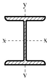
(بال‌ها و جان فشرده)
